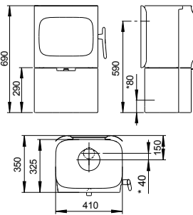
Jøtul F 105 B - con base
