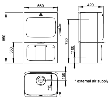
Jøtul F 305 B - base
