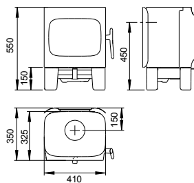
Jøtul F 105 SL - patas cortas
