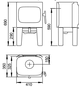
Jøtul F 105 LL - patas largas
