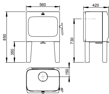
Jøtul F 305 LL - patas largas
